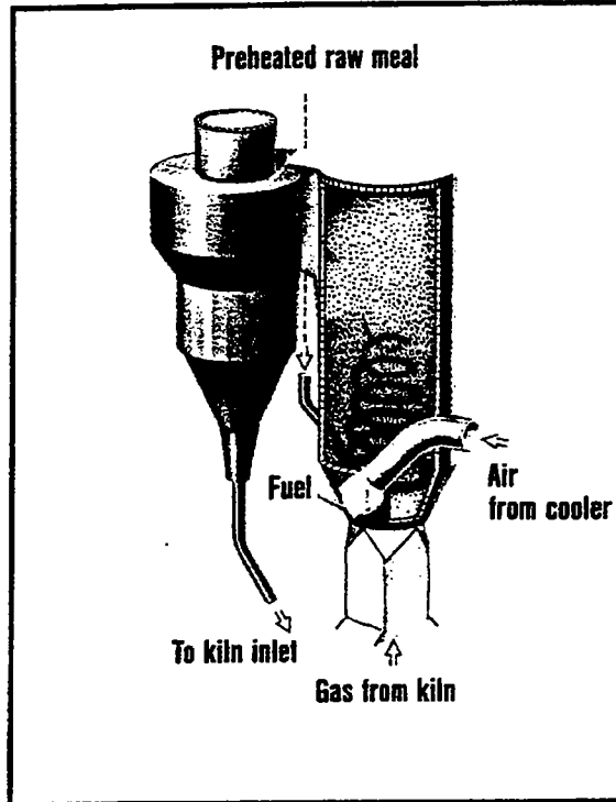
ILC calciner.
